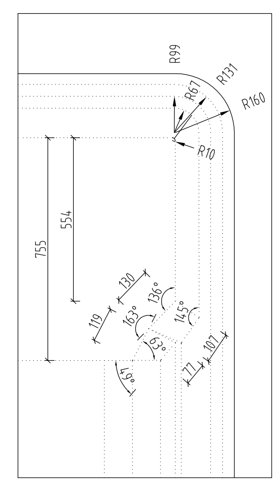
ROLLER NICHE DETAIL ROLLADEN NISCHE DETAIL DETAIL NIKY PRE ROLETU SCALE 1:10 MASSTABBE MIERKA
