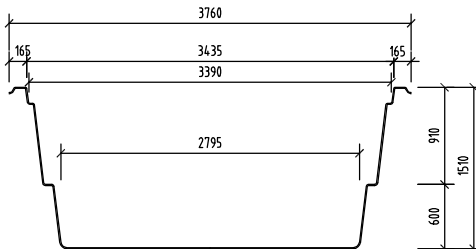
REZ 1 - 1 M 1:50
