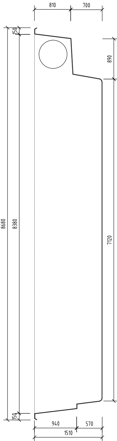
REZ 2 - 2 M 1:50 LONGITUDINAL SECTION QUERSCHNITT
